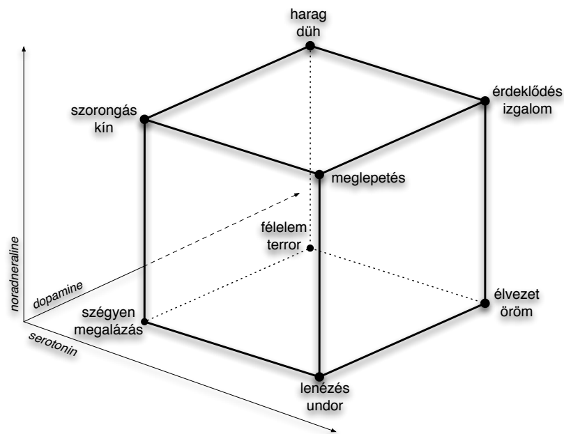
Figure 4.2: Lövhelm érzelmetipológiája
