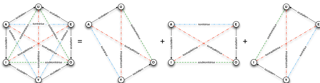
Figure 1.3: logikai hatszög és négyszögek
