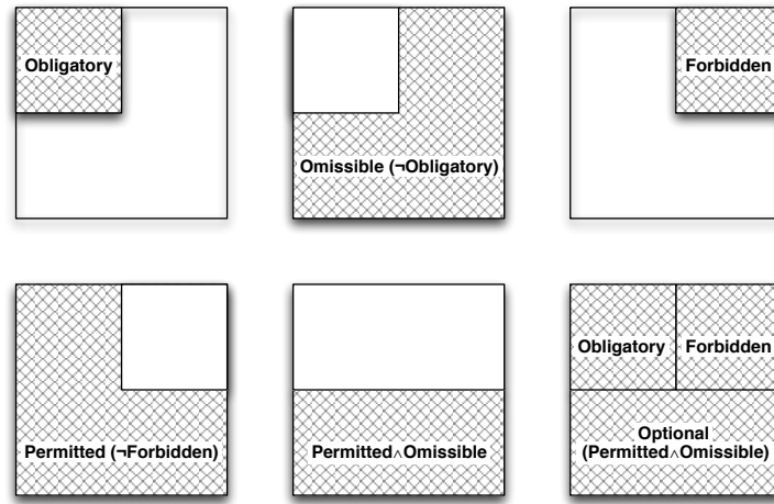
Figure 1.10: deontikus operátorok a JEPD elv szerint
