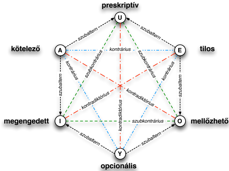
Figure 1.9: deontikus logikai hatszög
